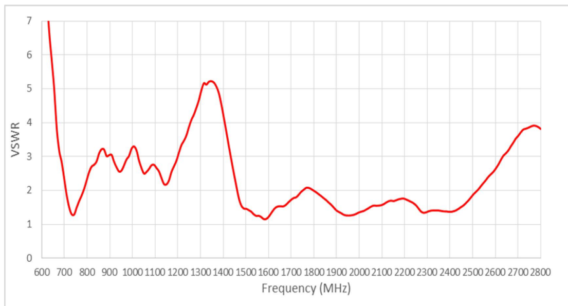
VSWR
